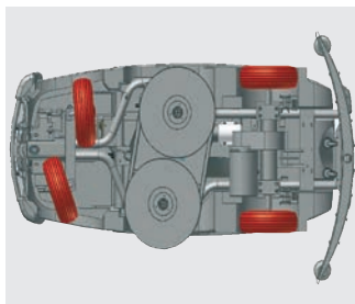
Kleiner Wendekreis durch fast 90° Radeinschlag
