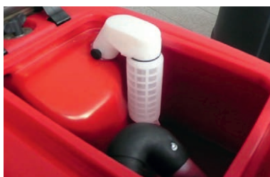
Effizienter Motorschutz dank Schwimmersystem
