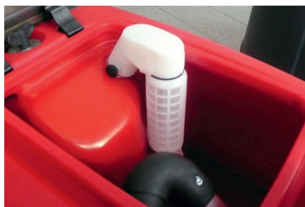
Effizienter Motorschutz dank Schwimmersystem
